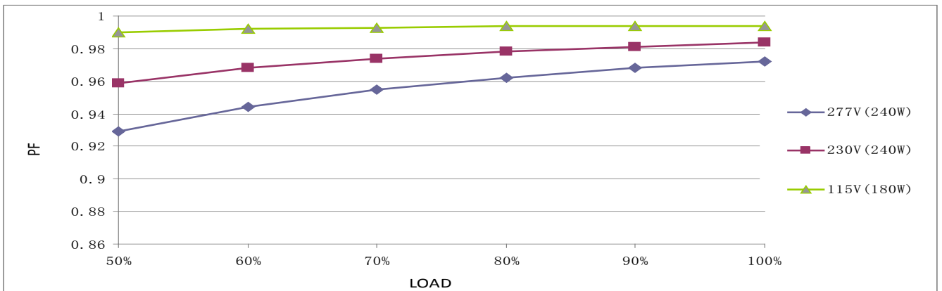
P.F vs LOAD
